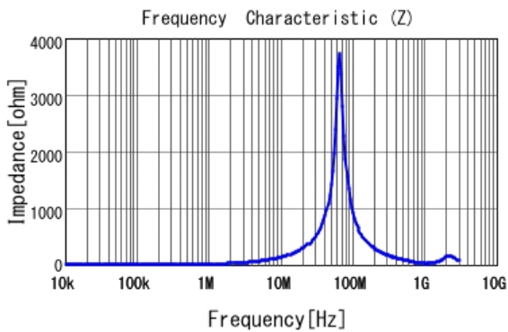
■ 1217AS-H-2R2N |Z|
