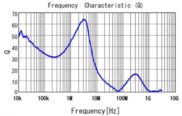
■ 1217AS-H-2R2N Q
