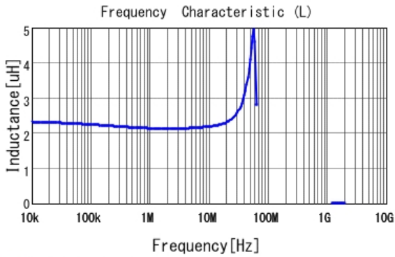
■ 1217AS-H-2R2N L
